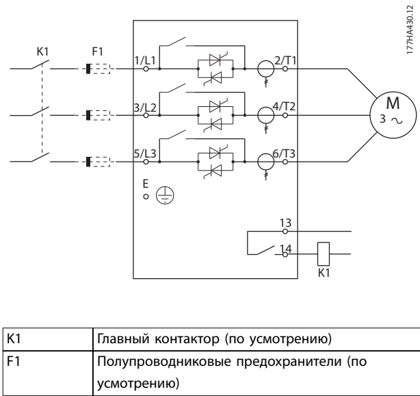
Рисунок 4.6 Линейный монтаж с внутренним шунтом
