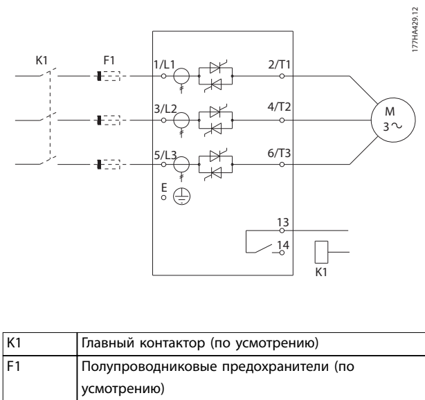
Рисунок 4.7 Линейный монтаж без шунта
