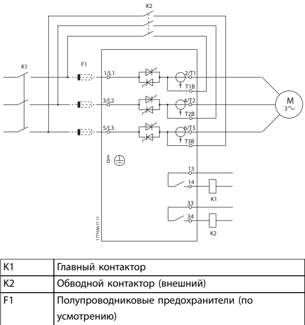
Рисунок 4.8 Линейный монтаж с внешним шунтированием, MCD5-0245C
