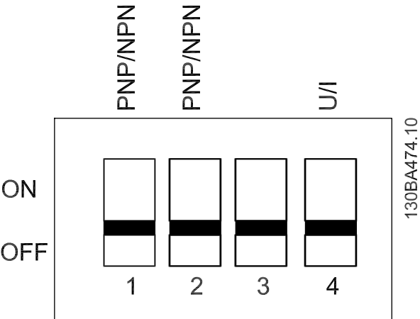
Рисунок 1.4 Переключатели S200, 1–4
