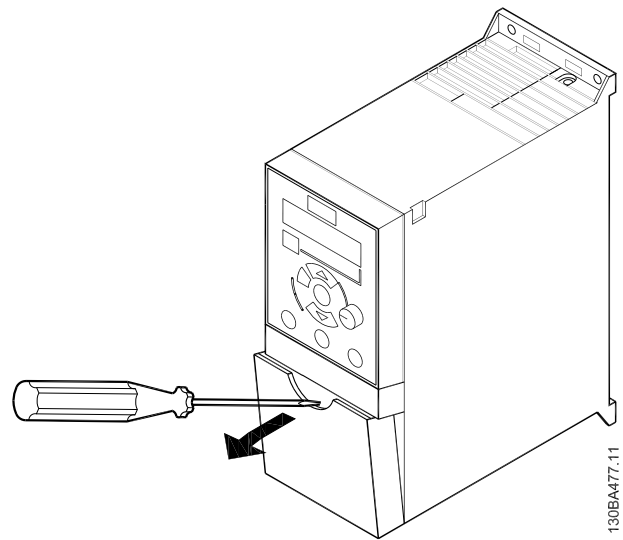
Рисунок 1.3 Снятие клеммной крышки
