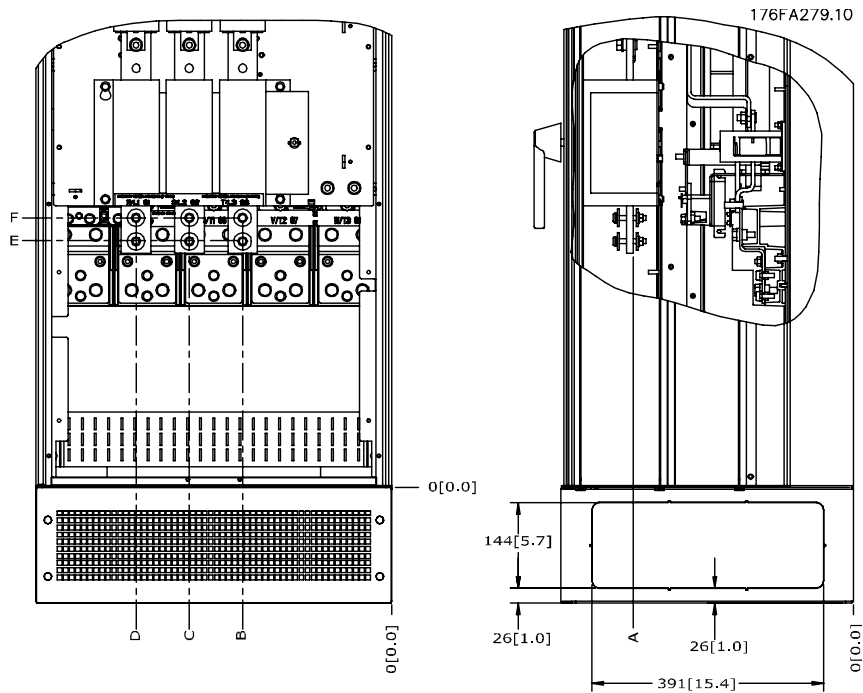
Рисунок 3.17: IP21 (NEMA type 1) и IP54 (NEMA type 12) расположение клемм электропитания корпуса
