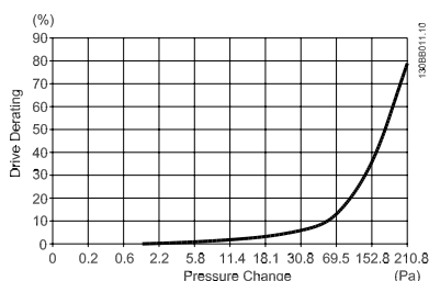
Рисунок 3.29: Корпус E Снижение значений относит. Изменение давления (Большой вентилятор), P315T5-P400T5 и P500T7-P560T7
