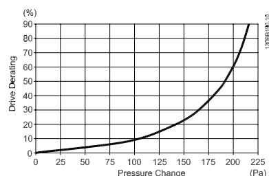
Рисунок 3.30: КорпусF1, F2, F3, F4 Снижение значений относит. Изменение давления
