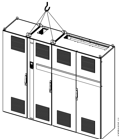
Рисунок 3.6: Рекомендуемый метод подъема, размер корпуса F4.
