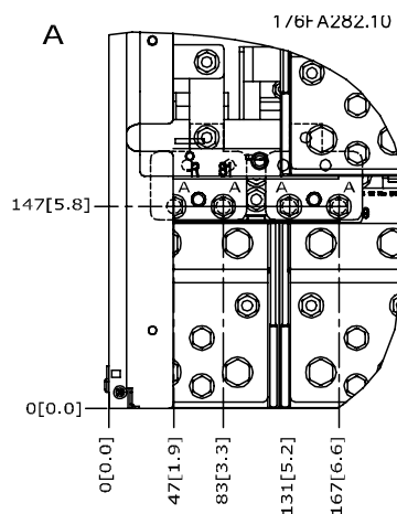
Рисунок 3.19: Расположение разъемов питания на корпусе IP00
