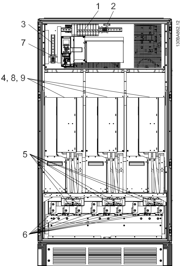
Рисунок 3.49: Шкаф инвертора, размер корпуса F2 и F4
