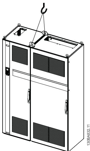
Рисунок 3.3: Рекомендуемый метод подъема, размер корпуса F1.
