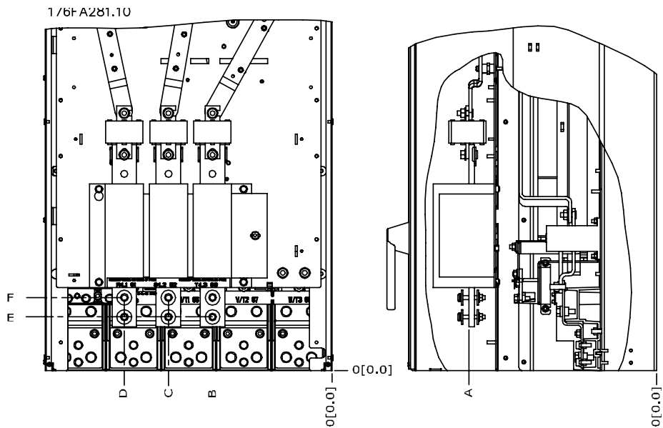
Рисунок 3.20: Расположение клемм электропитания корпуса IP00 с разъединителем
