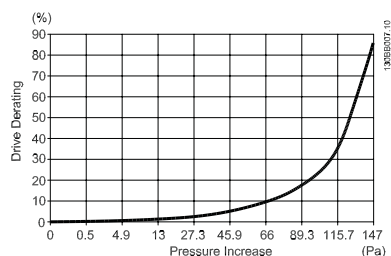
Рисунок 3.27: Корпус D Снижение значений относит. Изменение давления
