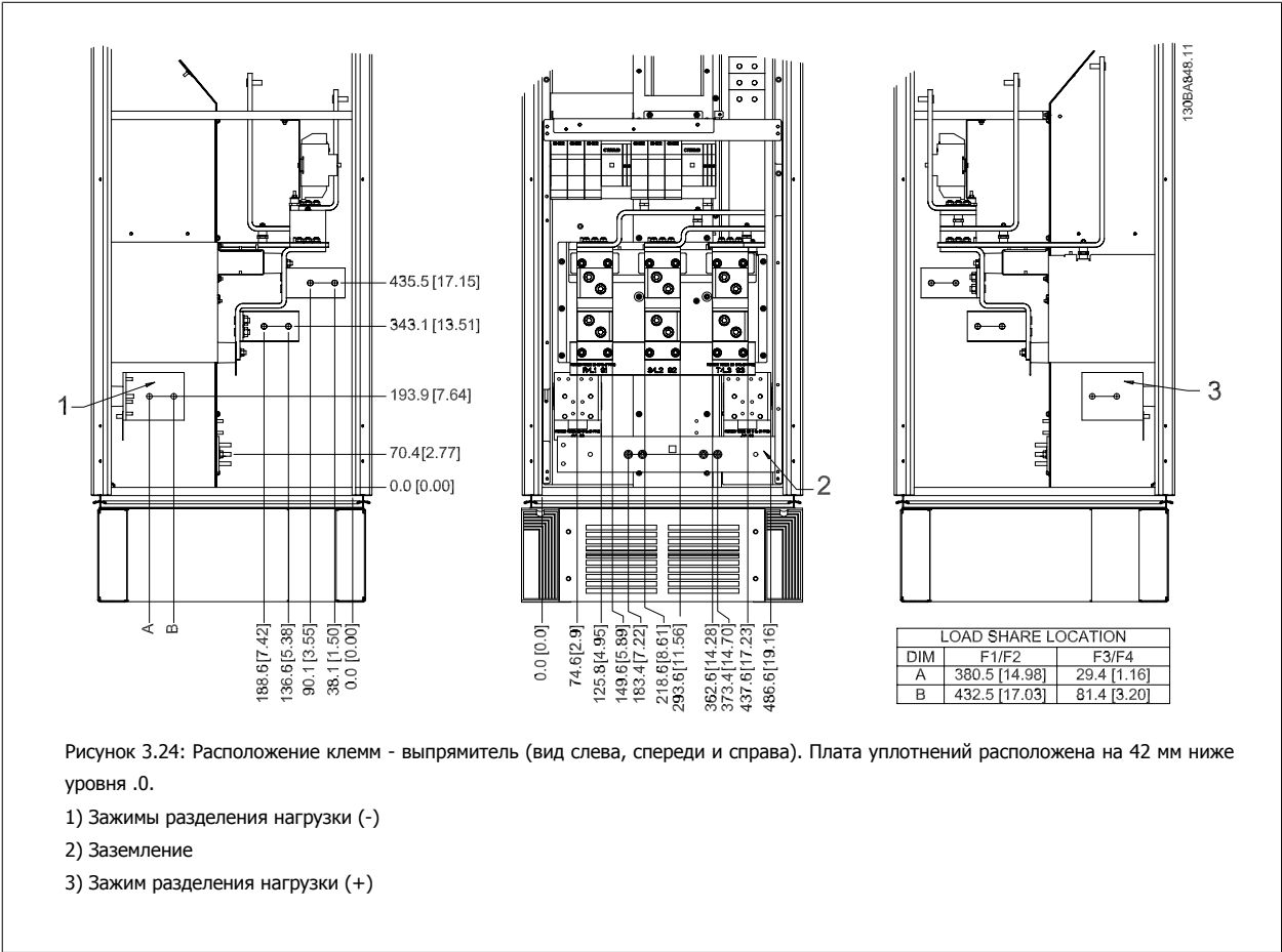
Расположение клемм - выпрямитель (F1, F2, F3 и F4)
