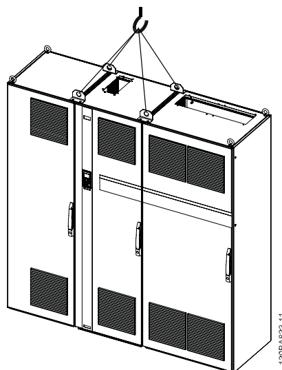
Рисунок 3.5: Рекомендуемый метод подъема, размер корпуса F3.
