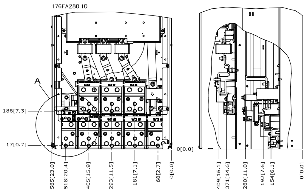
Рисунок 3.18: Расположение разъемов питания на корпусе IP00
