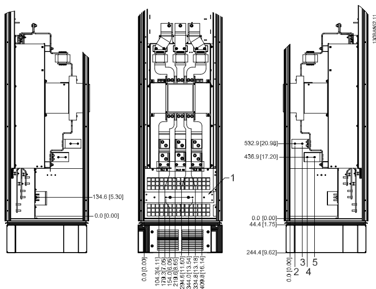
Рисунок 3.26: Расположение клемм - шкаф дополнительных устройств с автоматическим выключателем/выключателем в литом корпусе (вид слева, спереди и справа). Плата уплотнений расположена на 42 мм ниже уровня .0.
