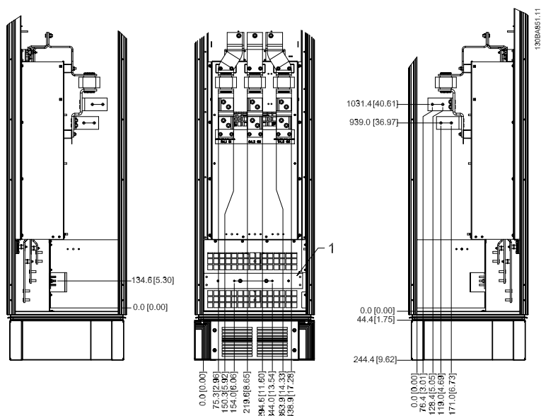
Рисунок 3.25: Расположение клемм - шкаф дополнительных устройств (вид слева, спереди и справа). Плата уплотнений расположена на 42 мм ниже уровня .0.
