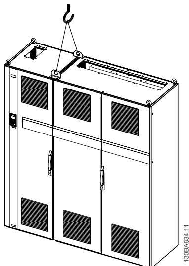
Рисунок 3.4: Рекомендуемый метод подъема, размер корпуса F2.
