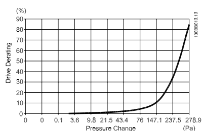
Рисунок 3.28: Корпус E Снижение значений относит. Изменение давления (Малый вентилятор), P250T5 и P355T7-P400T7
