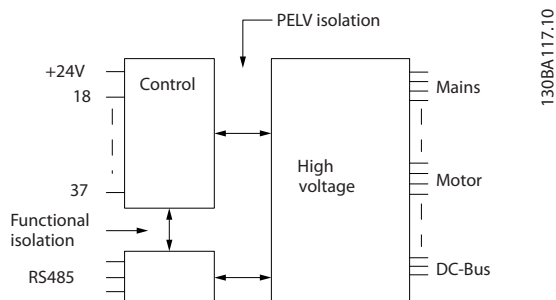
Рисунок 8.1 Изоляция PELV
