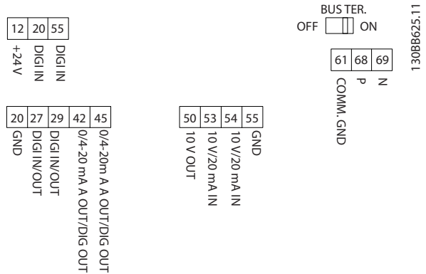
Рисунок 4.11 Клеммы управления
