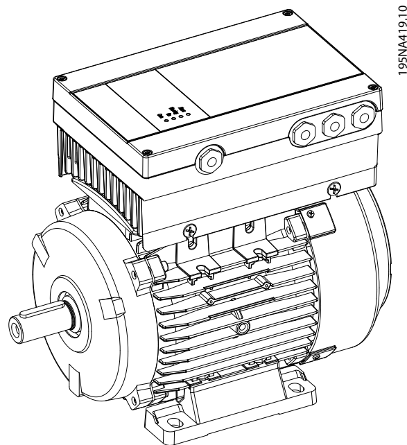
Рисунок 1.2 FCM 106
