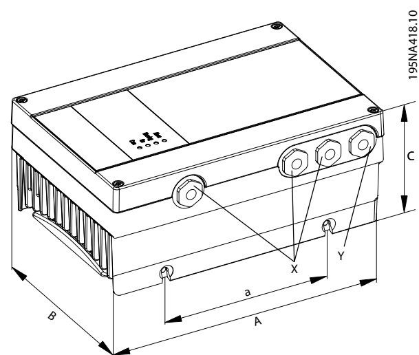
Рисунок 7.2 Размеры FCP 106
