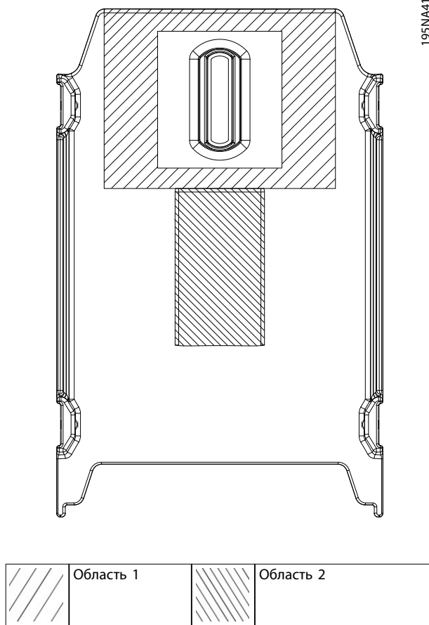
Рисунок 3.3 Крепежная пластина, руководство по сверлению отверстий
