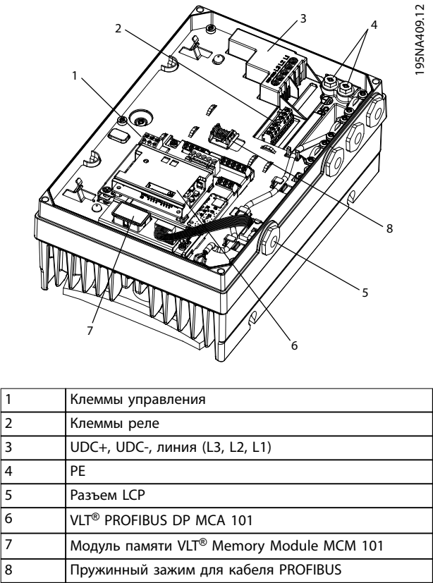
Рисунок 4.10 Расположение клемм и реле, МН2–МН3
