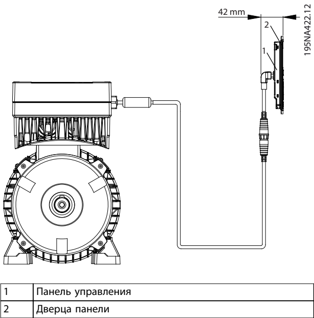
Рисунок 5.3 Дистанционный монтаж LCP
