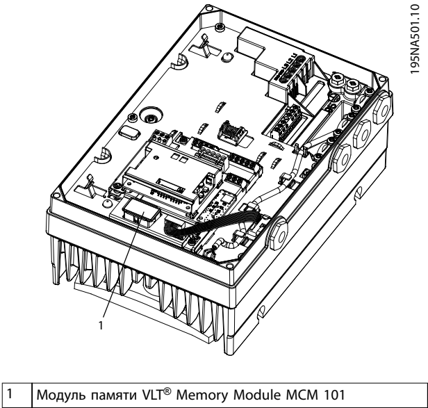
Рисунок 5.4 Расположение модуля памяти
