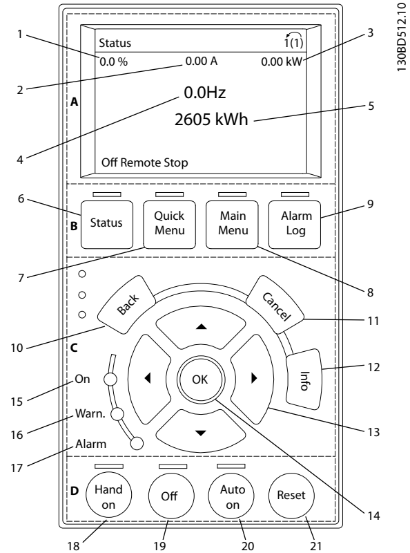
Рисунок 5.2 Панель местного управления (LCP)
